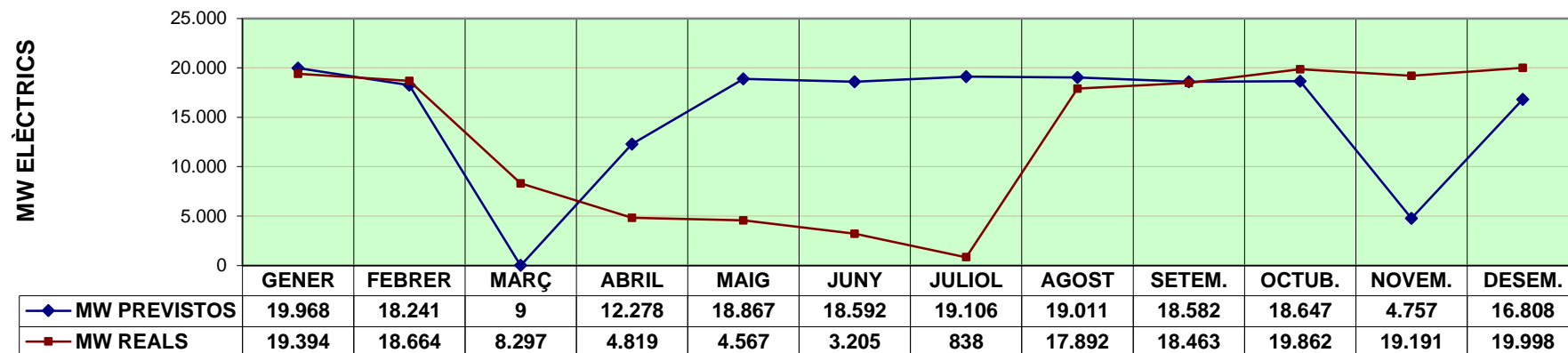
MW ELÈCTRICS PRODUIÏTS PREVISTOS I REALS MENSUALS
