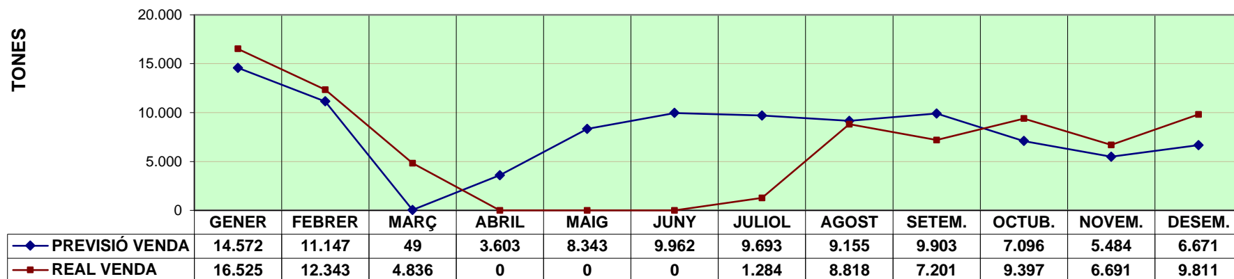
T. VAPOR VENUT PREVIST I REAL DISTRICLIMA
