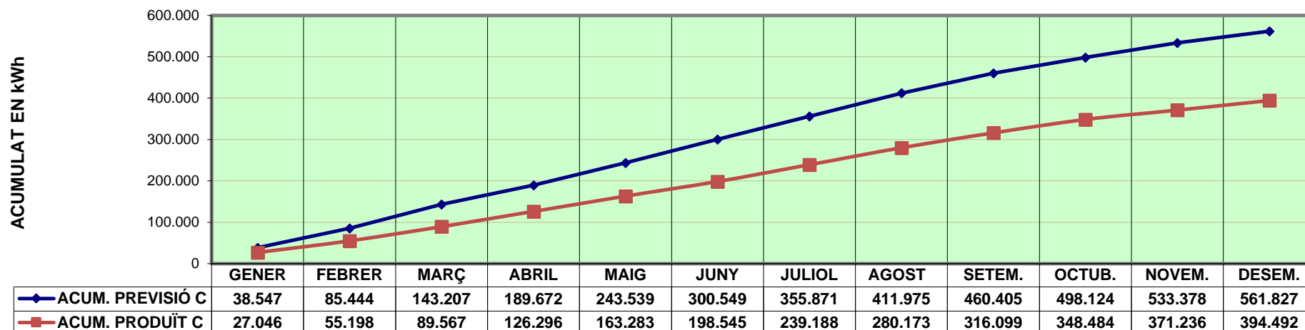
ACUMULATS DE PREVISIÓ I REAL DE PRODUCCIÓ FOTOVOLTAICA DEL FÒRUM GRUP C
