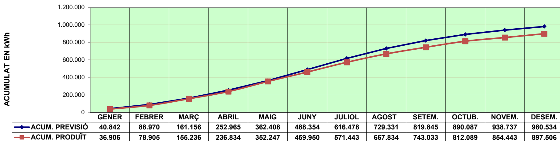
ACUMULATS DE PREVISIÓ I REAL DE PRODUCCIÓ FOTOVOLTAIQUES GRUP A+B+D
