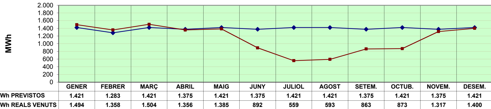
ENERGIA VENUDA A XARXA (MWh)
