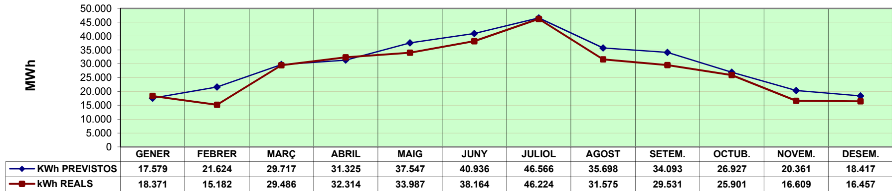
PRODUCCIÓ FOTOVOLTAIQUES D'AUTOGENERACIÓ (kWh)
