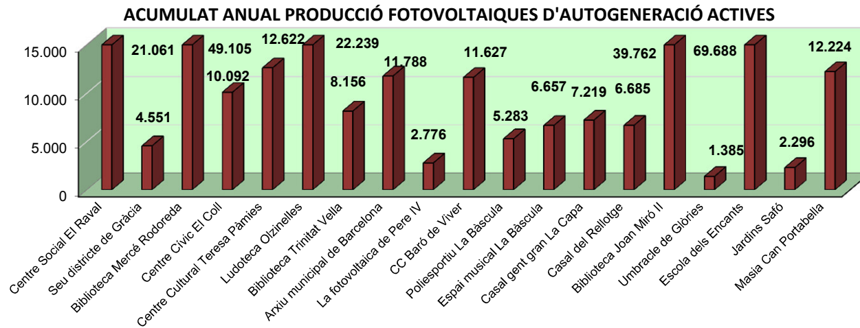
PRODUCCIÓ FOTOVOLTAIQUES D'AUTOGENERACIÓ (kWh)
