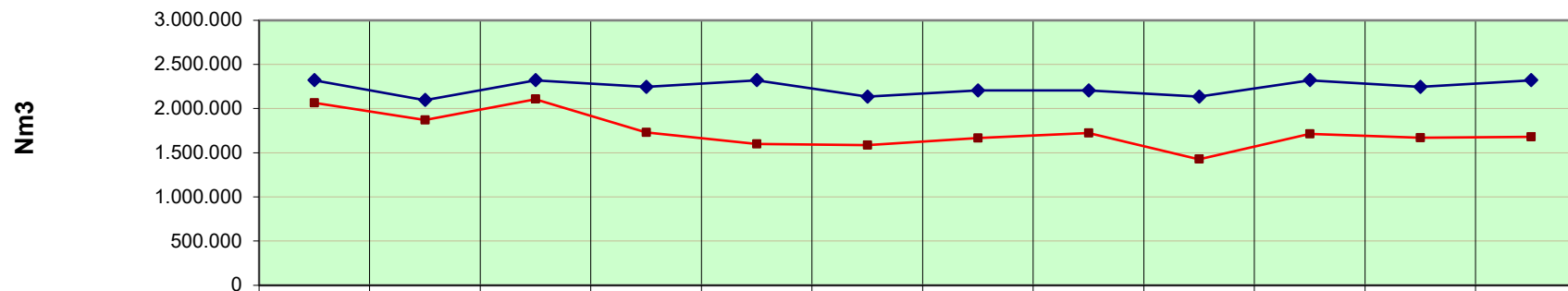
BIOGÀS A MOTORS (Nm3)
