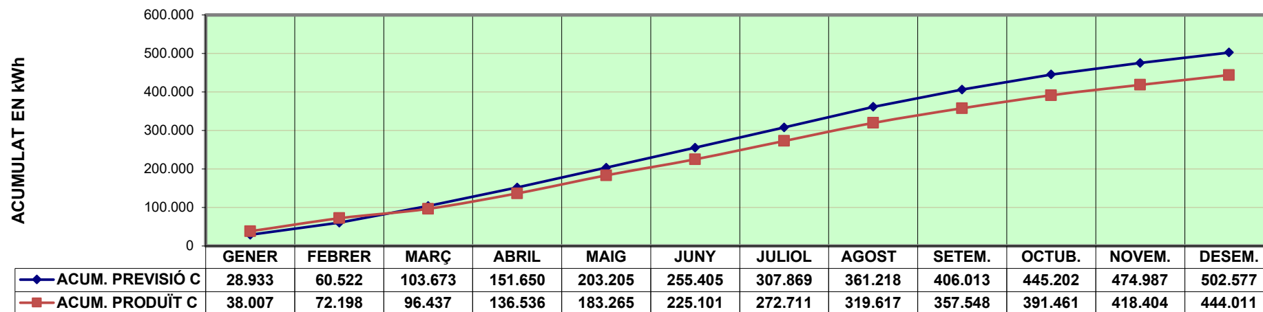
ACUMULATS DE PREVISIÓ I REAL DE PRODUCCIÓ FOTOVOLTAICA DEL FÒRUM GRUP C
