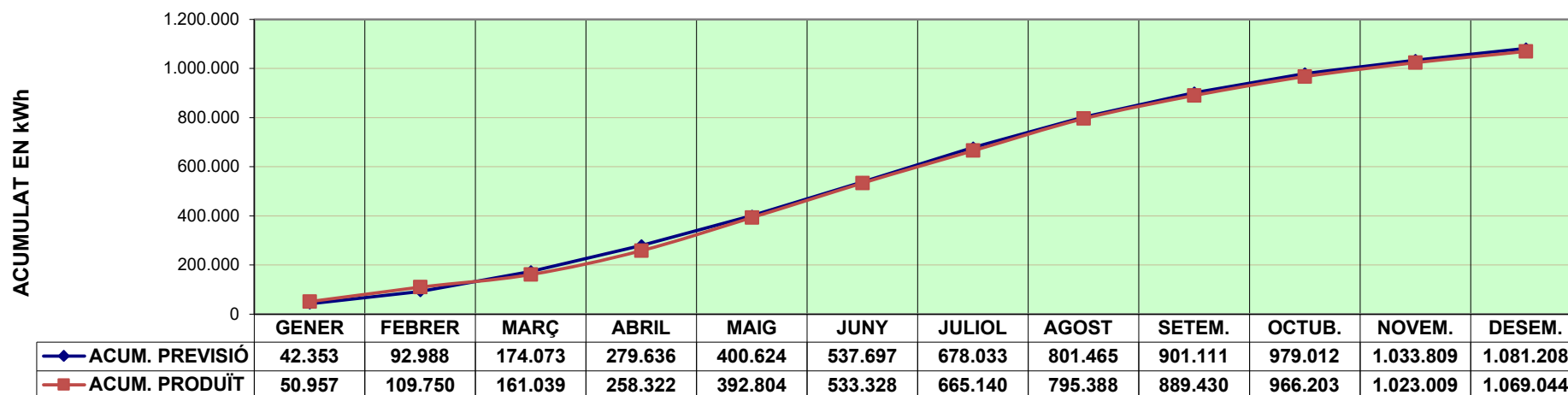
ACUMULATS DE PREVISIÓ I REAL DE PRODUCCIÓ FOTOVOLTAIQUES GRUP A+B+D
